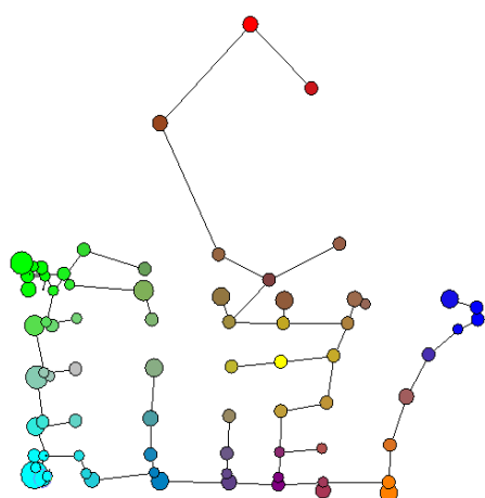
Рис. 1. Результаты ординации в отображении Сэммона
