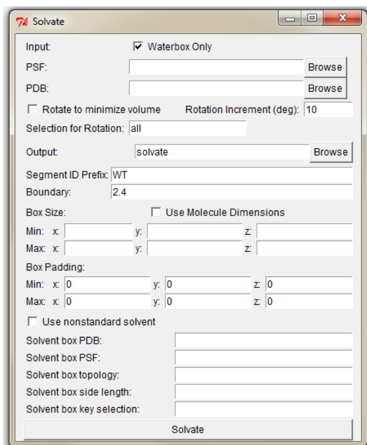
Рис. 7 Окно Solvate.
